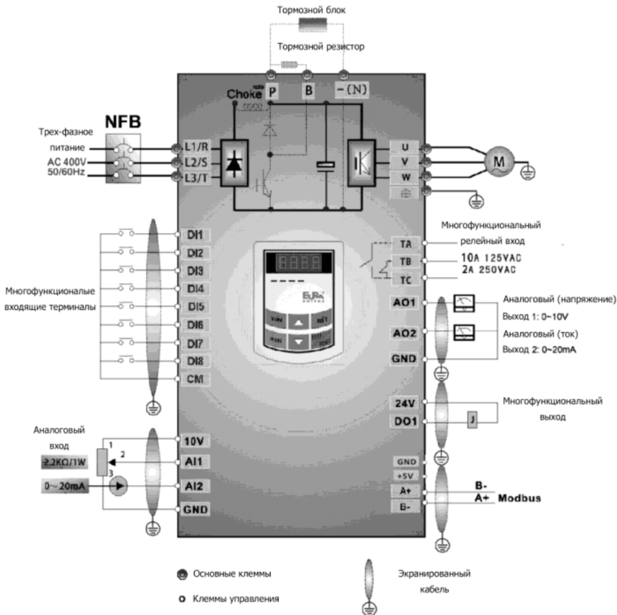
Стандартная схема подключения для многоскоростного управления (тип NPN)
