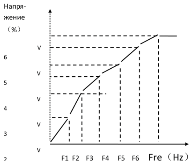
Рис 6-4 Полигональная линия Режим V/F
