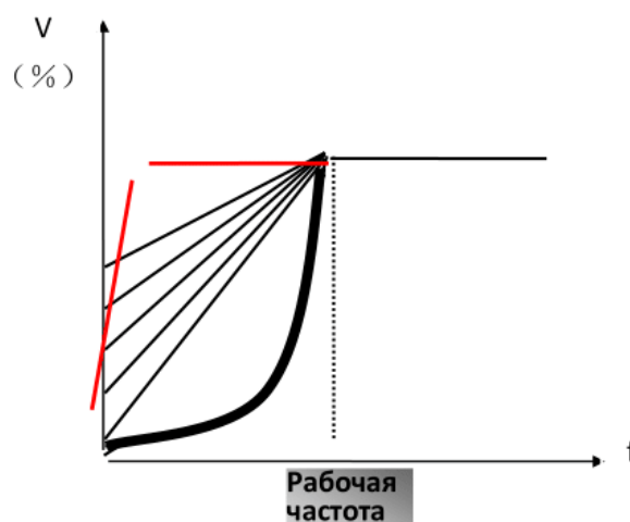
рис 6-3 Компенсация крутящего момента
