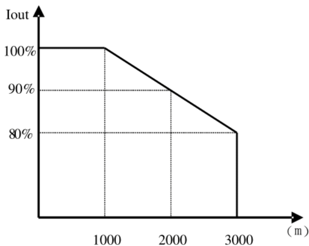
Рис. 1-1 Потеря мощности привода в зависимости от высоты
