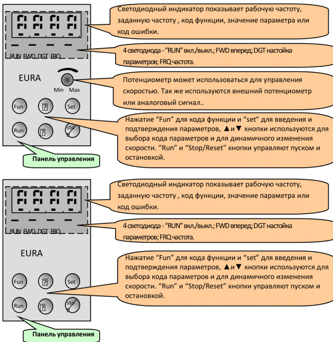
Рис.2-1 Панель управления
