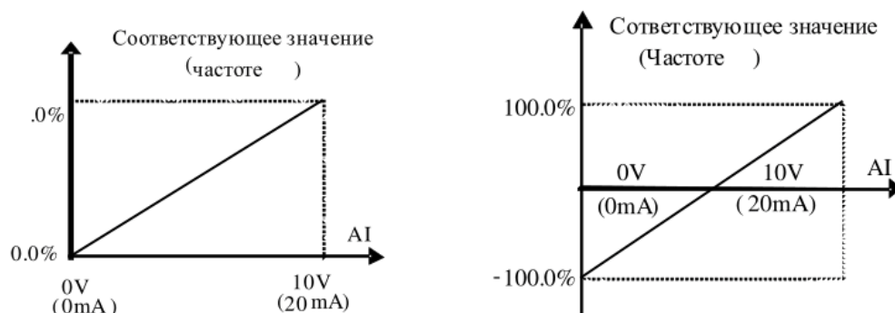
Рис. 6-13 Соответствие частоты аналоговому сигналу
