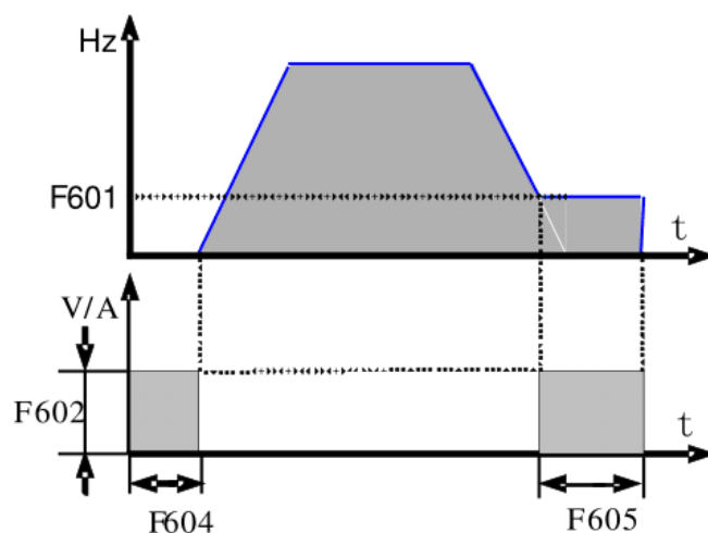
Рис. 6-19 DC торможение
