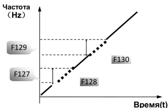
Рис. 6-2 Частота пропуска
