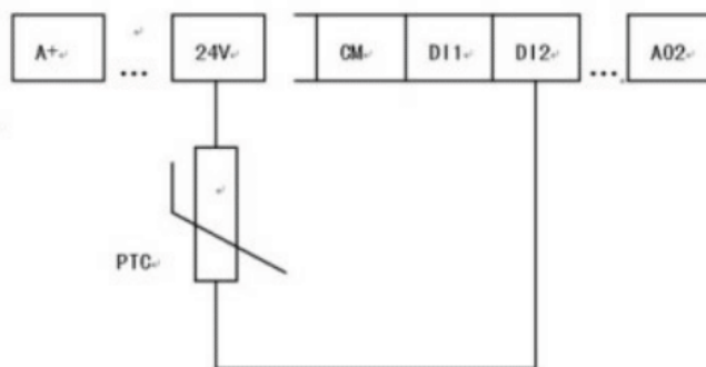
Рис. 6-6 PTC термозащита
