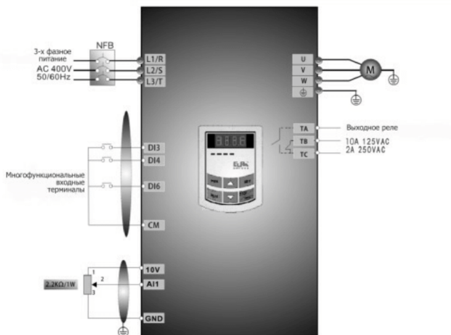
Рис. 5-3 Схема подключения 3
