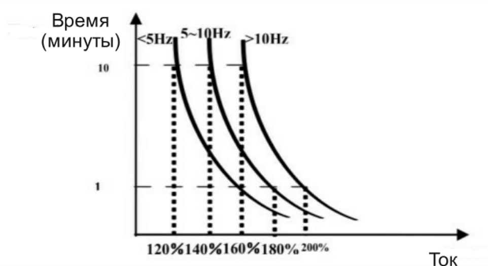
Рис 6-21 Значение защиты перегрузки двигателя
