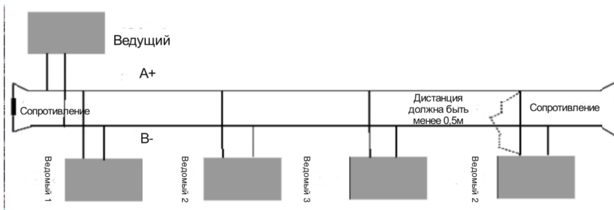
Схема подключения сопротивления
