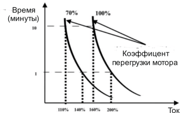
Рис. 5-19 Коэффициент перегрузки мотора
