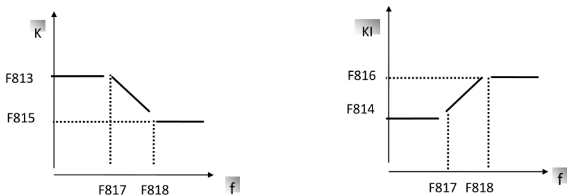
Рис. 6-22 параметр PID
