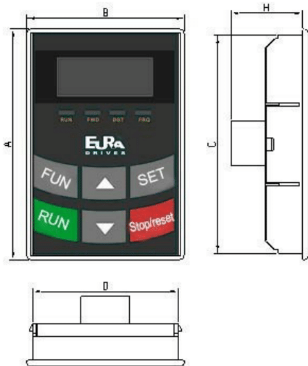
Чертеж панели
