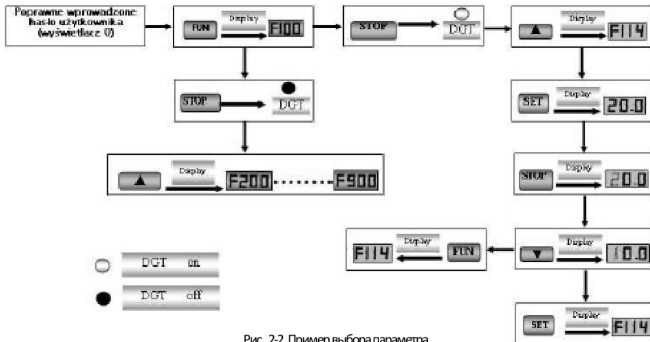
Рис. 2-2 Пример выбора параметра
